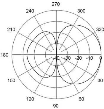
E-Plane | 166 MHz
